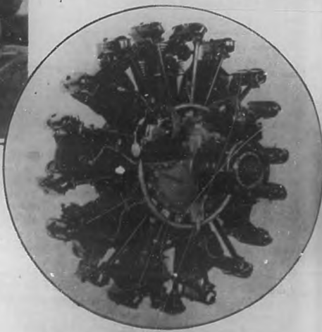
La foto muestra el motor "Whirlwind" de nueve cilindros y 225 caballos de fuerza, del monoplano "Espíritu de San Luis", usado por el capitán Lindbergh, para realizar su descomunal hazaña aviatoria.
