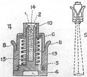
Diseño de la punta marcadora "Cuba".
